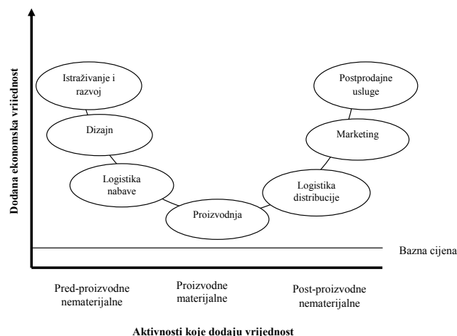
Slika 24. Lanac vrijednosti
